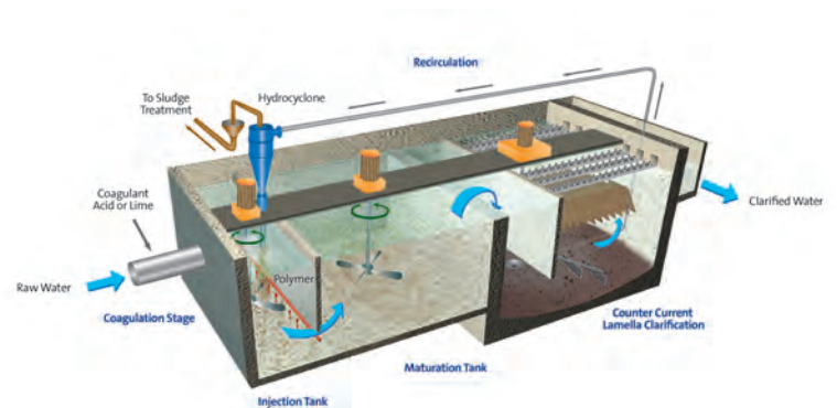
The Actiflo® Process
